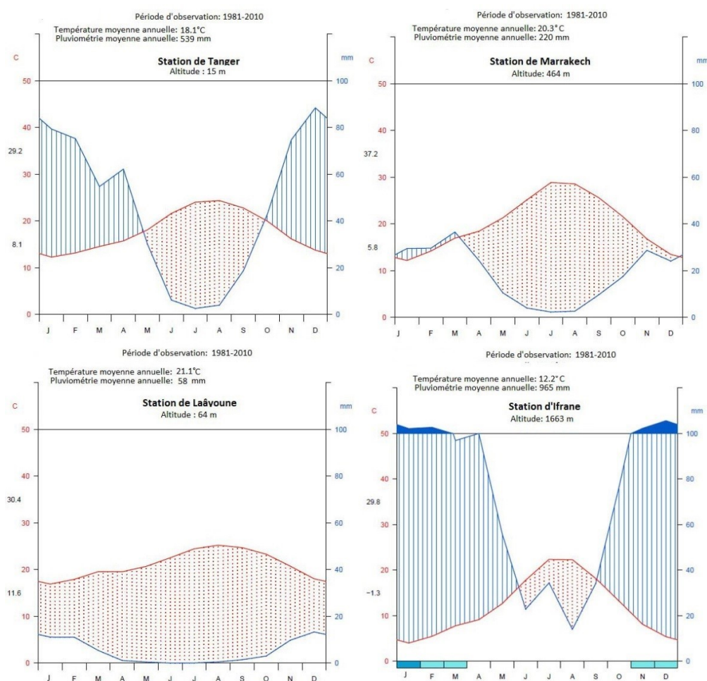
Figure 6. Diagrammes ombrothermiques selon l'indice de Gaussen-Bagnouls. Stations de Tanger (climat méditerranéen à été sec de type Cs), Marrakech (climat steppique de type BSh), Laâyoune (climat désertique de type BWh) et d'Ifrane (climat montagnard méditerranéen de type Ds). Pour le diagramme d'Ifrane, sur l'axe horizontal des mois, les cases en bleu indiquent les Tmin extrêmes en dessous de 0°C. (Le seuil de 100 mm est dépassé pendant les mois froids). [Source : © Hanchane]
